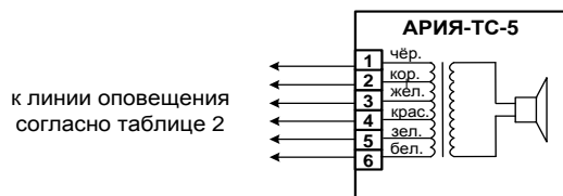
Рис. Схема подключения
