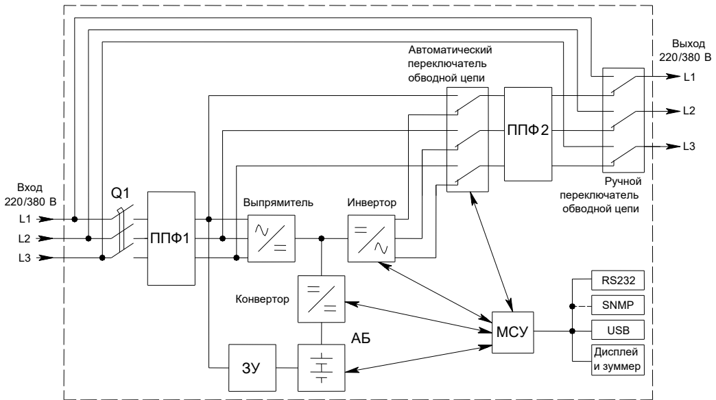
Рисунок 1 - Структурная схема ИБП
