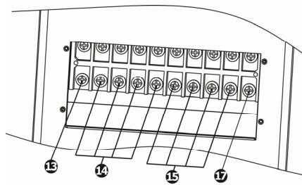
Рисунок 7 - Вид клеммных блоков на задней панели ИБП ATS 30000 3/3 T-BX, ATS 30000 3/3 T-X
