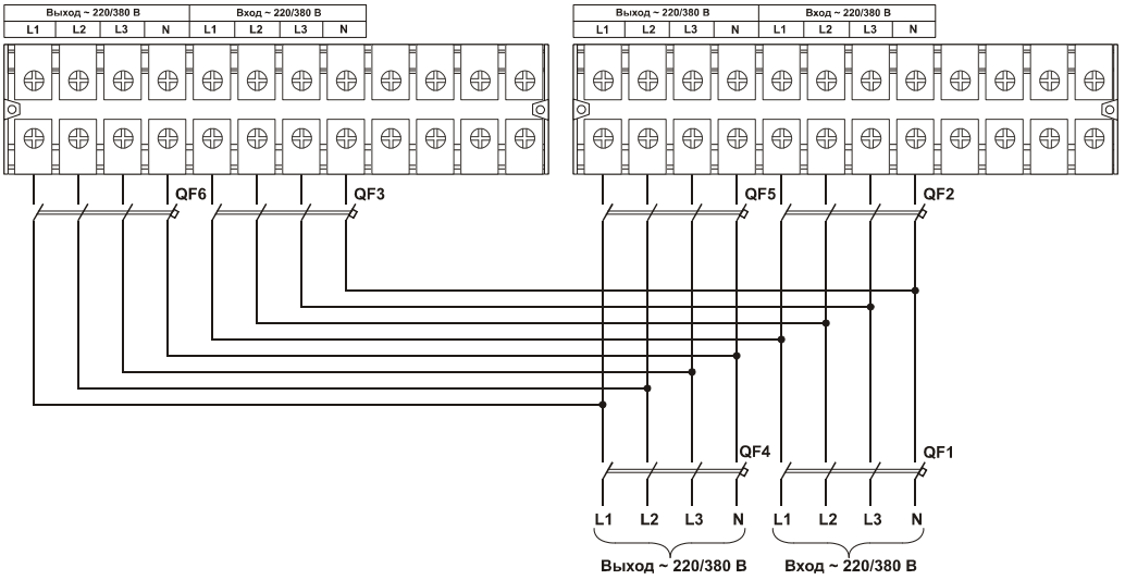
Рисунок 28 – Соединение входов и выходов двух ИБП в параллельной системе
