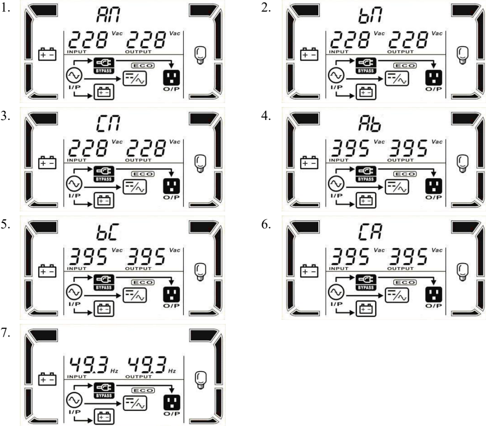
Рисунок 22 – Показания LCD-дисплея ИБП в режиме экономии энергии
