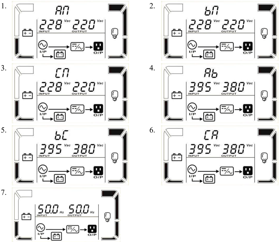
Рисунок 18 – Показания LCD-дисплея ИБП в дежурном режиме
