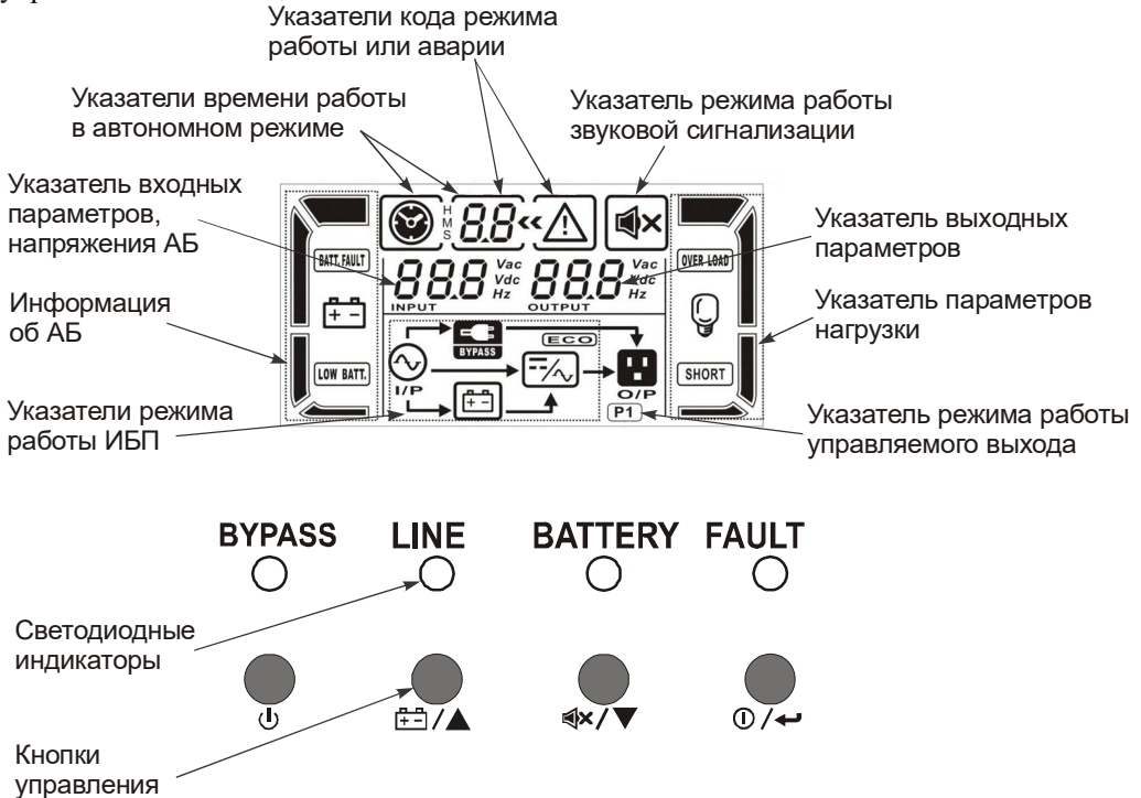
Рисунок 2 – Внешний вид органов управления и индикации ИБП
