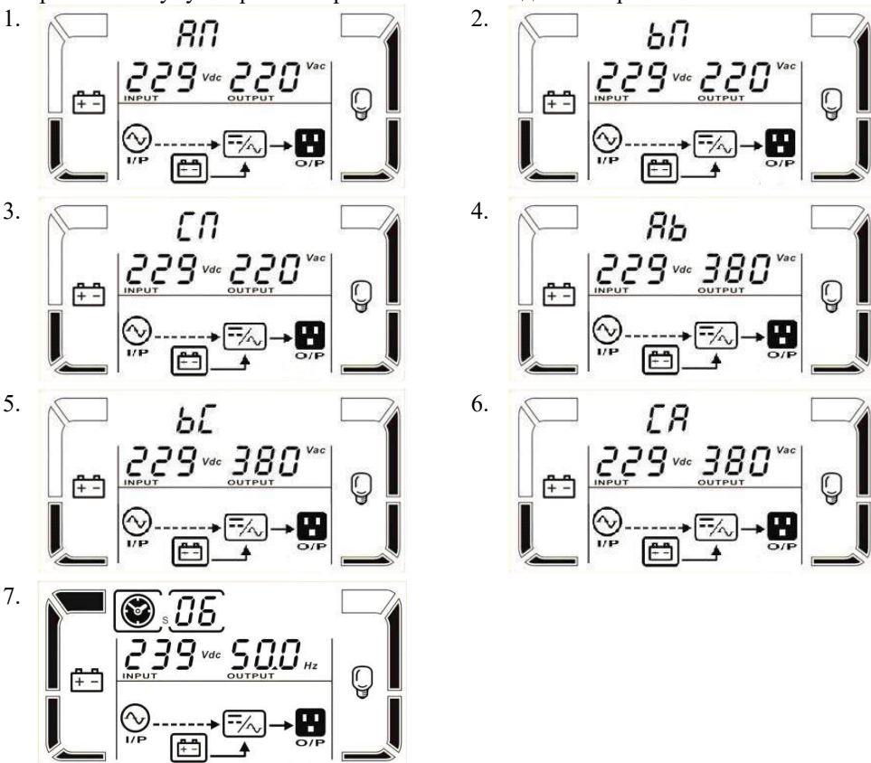
Рисунок 21 – Показания LCD-дисплея ИБП в режиме тестирования батарей
