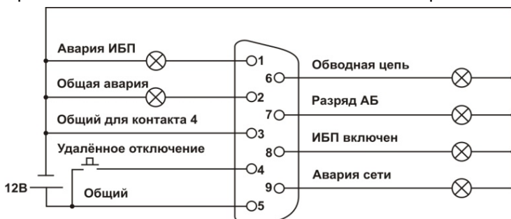
Рисунок 13 – Электрическая схема организации контроля и управления ИБП с электропитанием от источника постоянного тока напряжением +12 В
