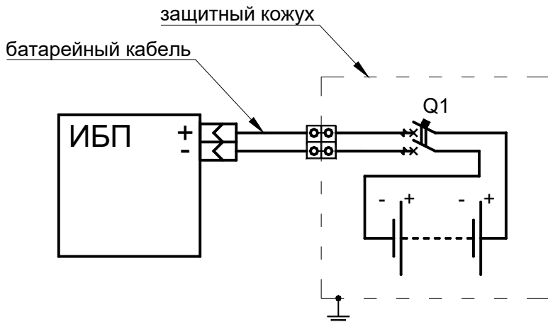
Рисунок 10 – Схема электрическая подключения аккумуляторов к ИБП
