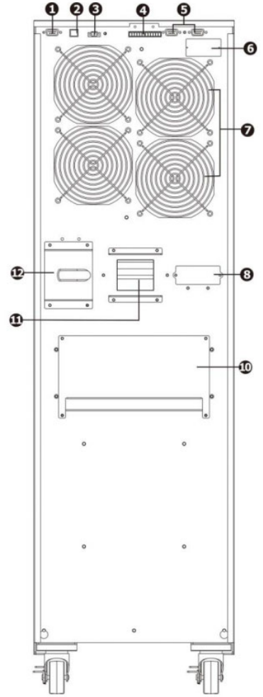
Рисунок 5 - Задняя панель ИБП ATS 30000 3/3 T-X
