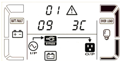
Рисунок 23 – Показания LCD-дисплея ИБП с кодами предупреждающих сообщений
