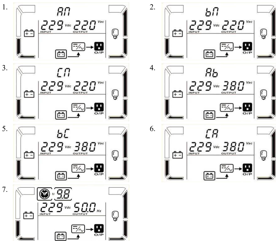
Рисунок 19 – Показания LCD-дисплея ИБП в автономном режиме
