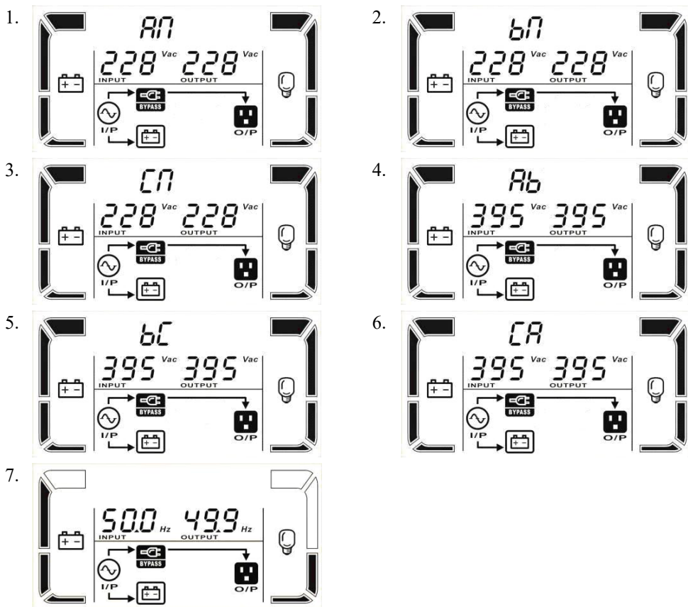
Рисунок 17 – Показания LCD-дисплея в режиме работы ИБП по встроенной обходной цепи
