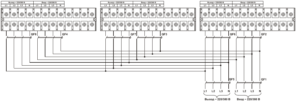
Рисунок 29 – Соединение входов и выходов трех ИБП в параллельной системе
