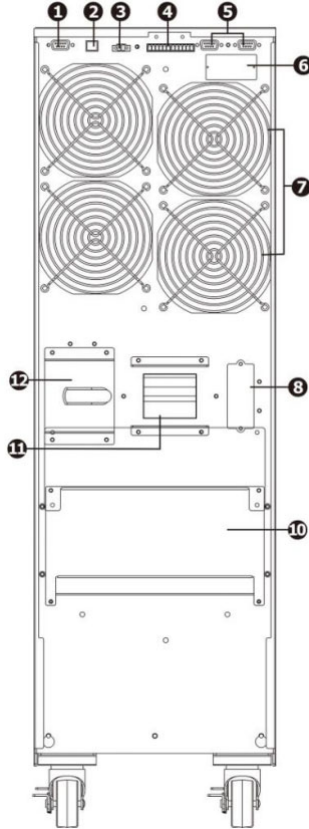
Рисунок 4 - Задняя панель ИБП ATS 30000 3/3 T-BX
