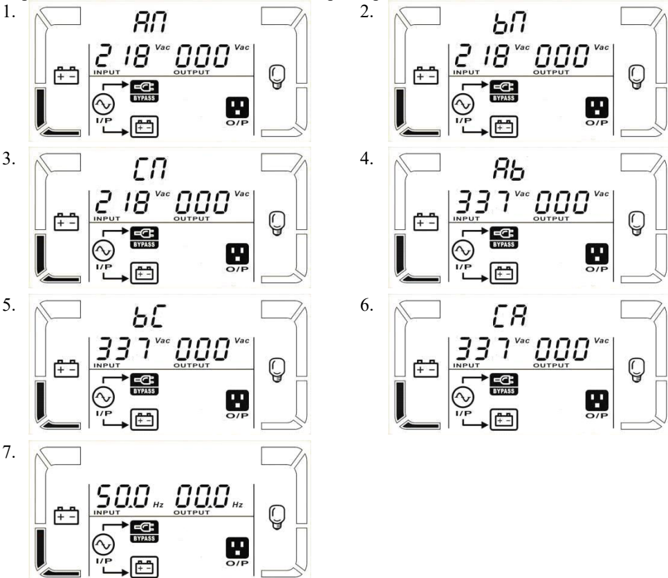
Рисунок 16 – Показания LCD-дисплея ИБП в режиме ожидания
