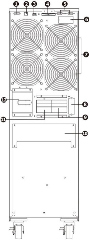
Рисунок 3 - Задняя панель ИБП ATS 10000 3/3 T-BX, ATS 10000 3/3 T-X, ATS 15000 3/3 T-BX, ATS 15000 3/3 T-X, ATS 20000 3/3 T-BX, ATS 20000 3/3 T-X
