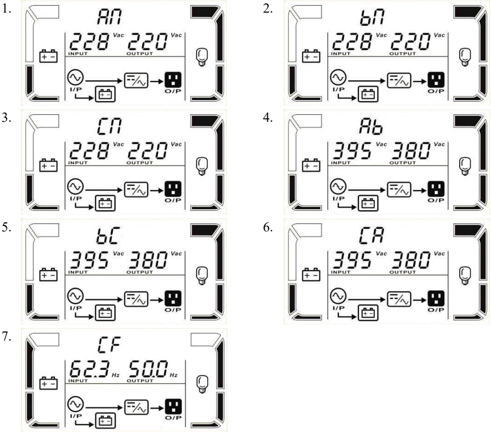
Рисунок 20 – Показания LCD-дисплея ИБП в режиме преобразователя частоты
