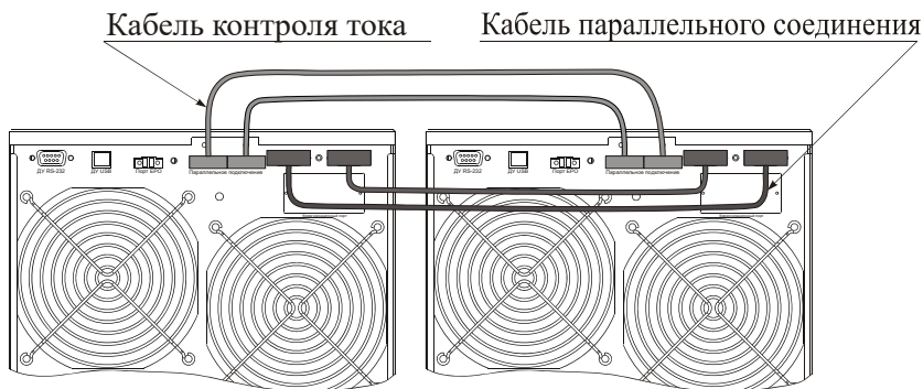
Рисунок 26 – Подключение информационных кабелей к двум ИБП в параллельной системе
