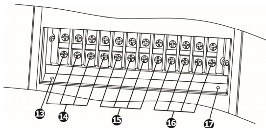
Рисунок 6 – Вид клеммных блоков на задней панели ИБП ATS 10000 3/3 T-BX, ATS 10000 3/3 T-X, ATS 15000 3/3 T-BX, ATS 15000 3/3 T-X, ATS 20000 3/3 T-BX, ATS 20000 3/3 T-X
