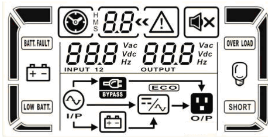
Рисунок 15 – Показания LCD-дисплея ИБП при включении
